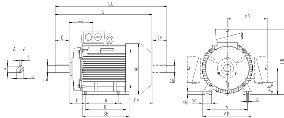
Outline Dimensions / Umriss Abmessungen
